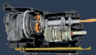
Plynulé převodové ústrojí od 0 do 50 km/h
